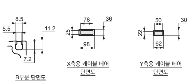
B부분 단면도
